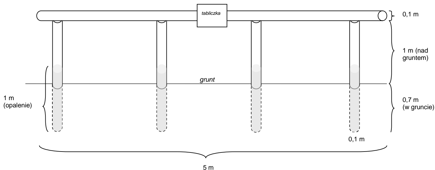
Szkic bariery
